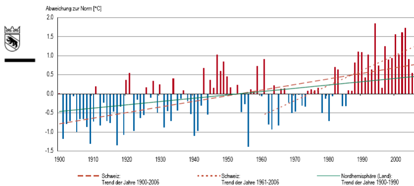
Abb. 17 > Jahresmitteltemperaturen in der Schweiz 1900–2006.
